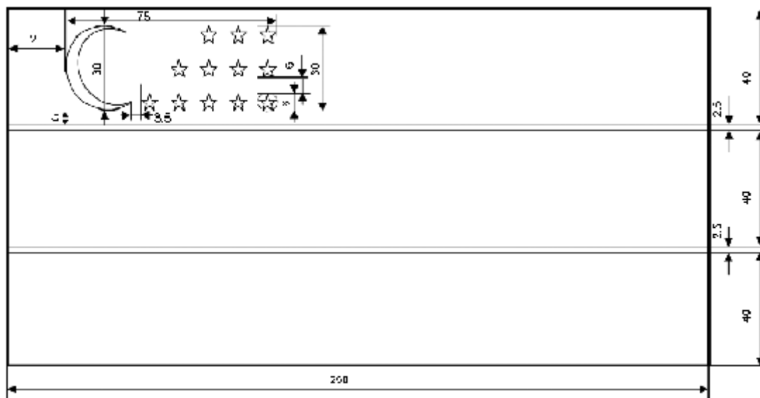
Sxematik rasmi
